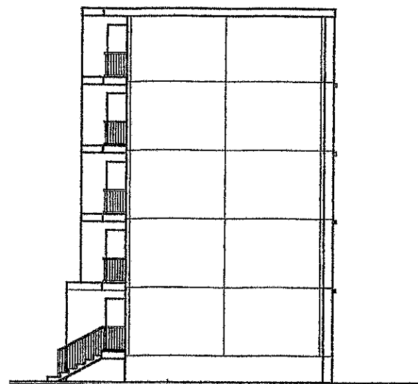
西側立面図
