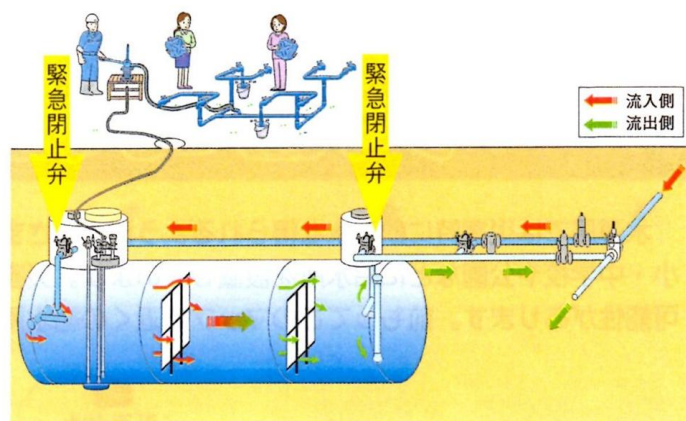
災害用地下給水タンク概要図
